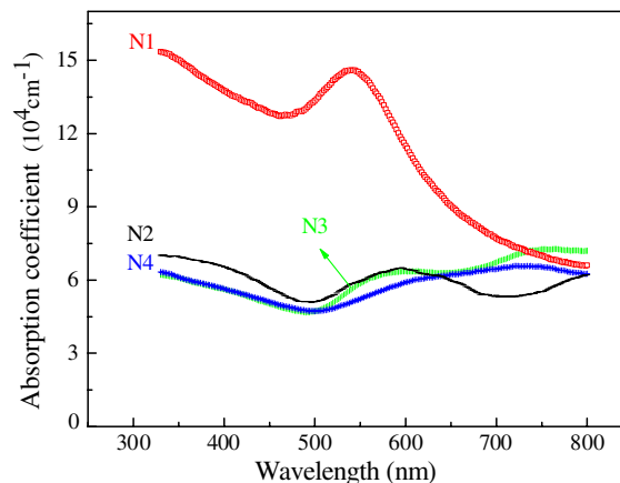
Figure 2. Optical absorption properties of the samples: (a) N1 (film, 12 nm); (b) N2 (array, 8 nm); (c) N3 (array, 14 nm); (d) N4 (array, 26 nm).
